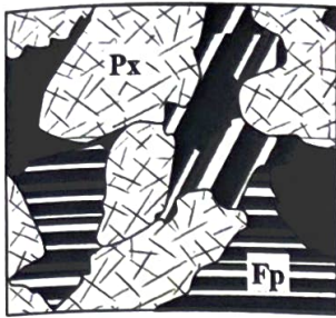
Gabbro
