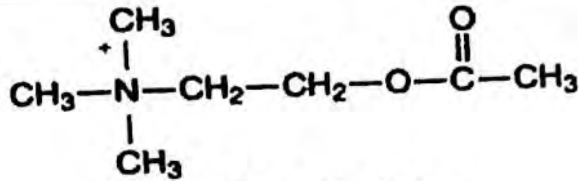
Acétylcholine
